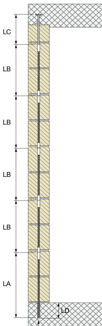
Eisen geklebt mit Injektionsmörtel ancoBOND® Armature scellée avec le mortier d'injection ancoBOND®
