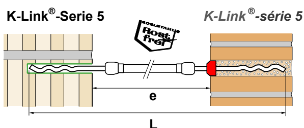
Sanierungsanker (inkl. eine Siebhülse) Ancre d'assainissement (1 tamis incl.)
