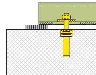
Befestigung mit Ankerschiene
