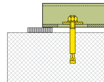
Befestigung mit Bolzenanker
