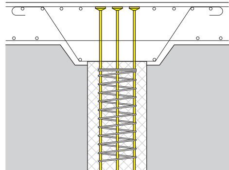
Pfeilkopfdetail in Fahrbahnplatte Encastrement de pieux d'une dalle de roulement
