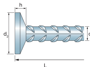
Typ 1 (ancoFIX®)
