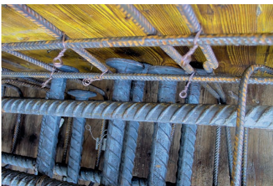
Verankerung mit ancoFIX®-Bewehrungen Ancrage avec l'armature ancoFIX®
