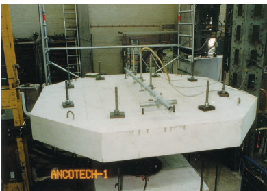
Zulassungsversuche Technische Universität München (D) (1991) Essais pour l'homologation Université tech- nique à Munich (D) (1991)
