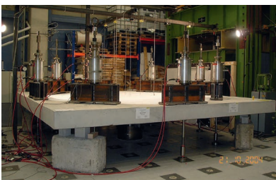
Grossversuche in Karlsruhe (2004) Campagne de recherche à Karlsruhe (2004)
