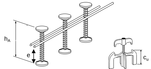
Durchstanz / Poinçonnement
