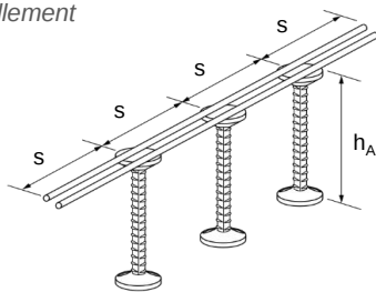
Schub / Cisaillement
