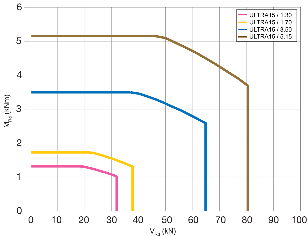
Interaktions Diagramm M_{Rd} / V_{Rd}
