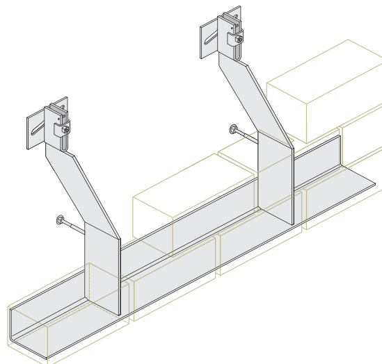
Winkelkonsolen AKO
