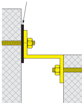
Thermische Trennung / Bande thermique
