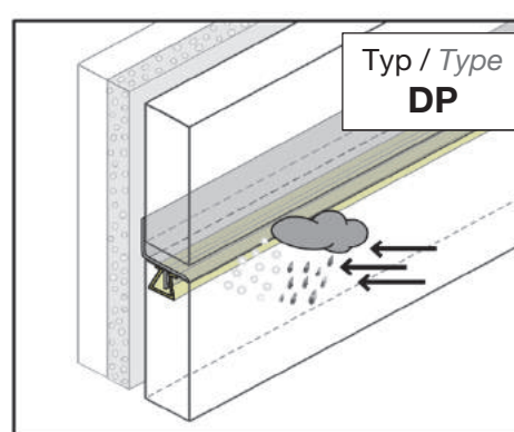
Fugenprofil horizontal Joint d'étanchéité horizontal
