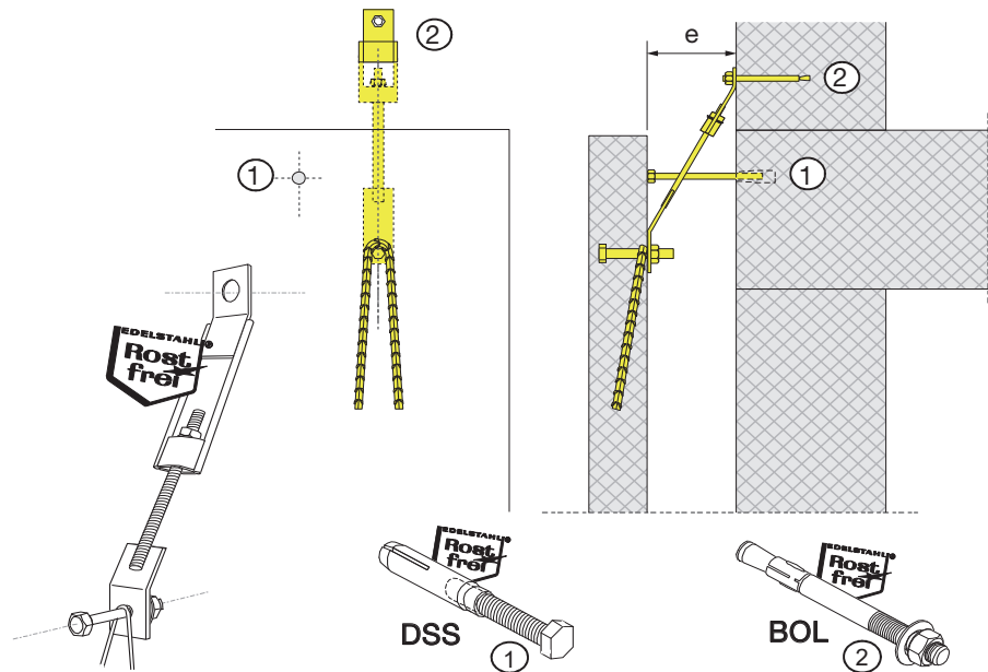
ATLAS® - Anker Ancre ATLAS®
