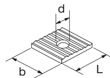
Zahnplatte Plaques crantées
