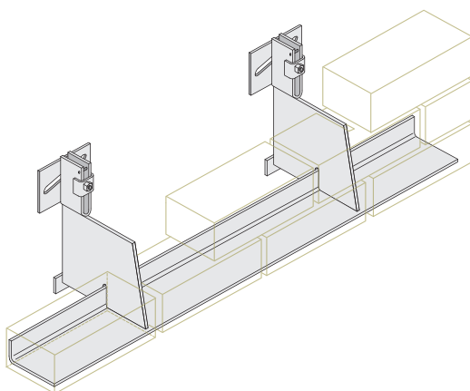
Abfangkonsolen AKN
