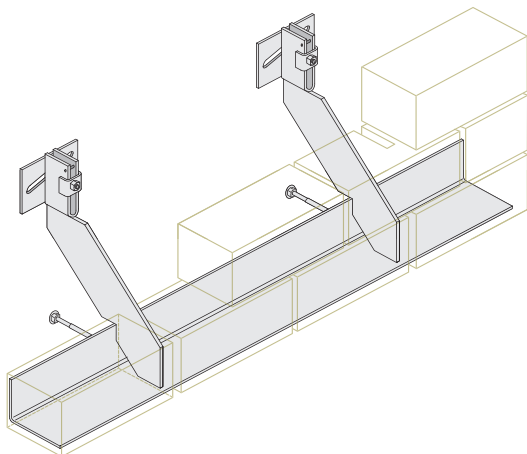
Abfangkonsolen AKL
