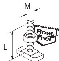
Hammerkopfschrauben Boulon à tête marteau
