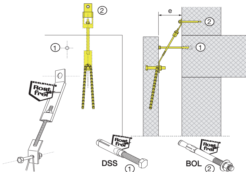
ATLAS® - Anker Ancre ATLAS®
