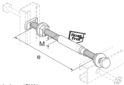
Spannverbindung 'SVA'
