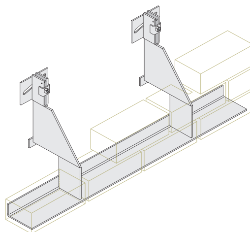
Winkelkonsolen AKO
