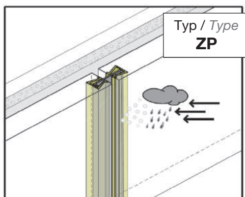
Fugenprofil vertikal Joint d'étanchéité vertical
