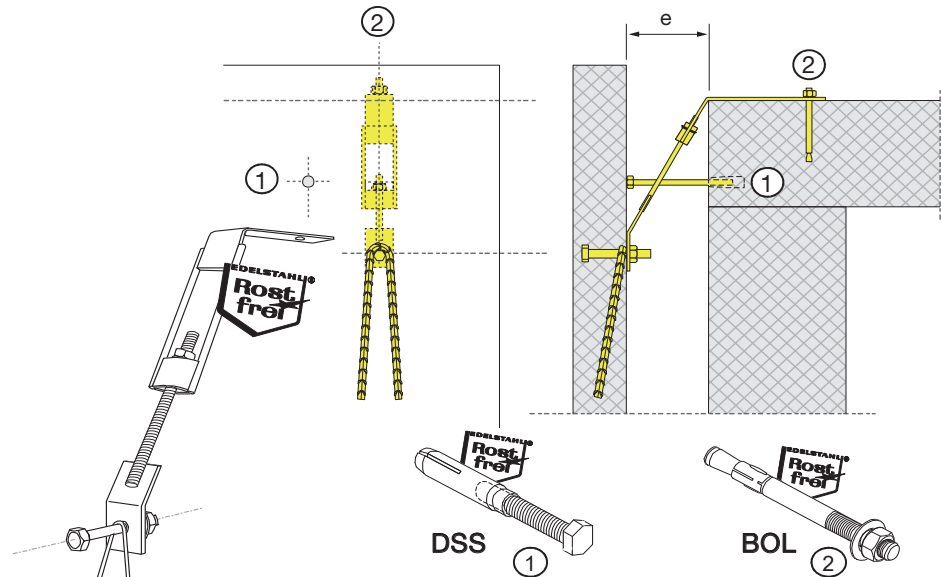
ATLAS® - Anker Ancre ATLAS®
