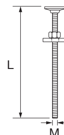
Typ / Type C
