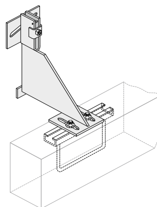
Winkelkonsolen AKM
