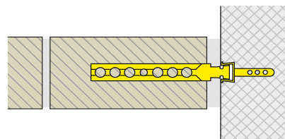
Maueranschluss mit ML-Anker (S.90) Liaison de murs avec ancre ML (p.90)
