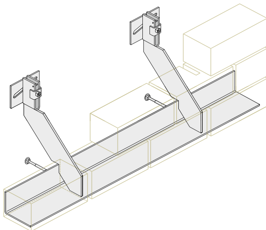
Abfangkonsolen AKL
