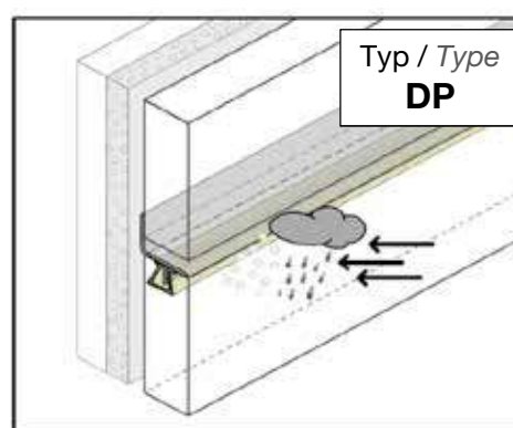
Fugenprofil horizontal Joint d'étanchéité horizontal
