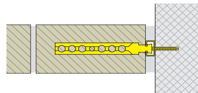
Maueranschluss mit ML-Anker (S.82) Liaison de murs avec ancre ML (p.82)
