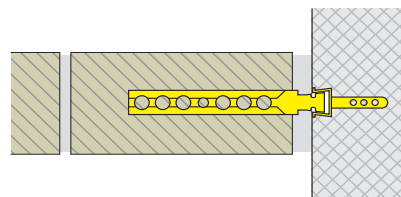
Maueranschluss mit ML-Anker (S.82) Liaison de murs avec ancre ML (p.82)
