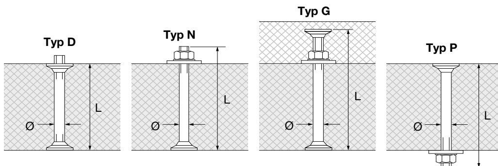
ancoSAN®-Durchstanz-Sanierungsanker
