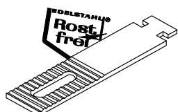
Zahnlasche Connecting plates
