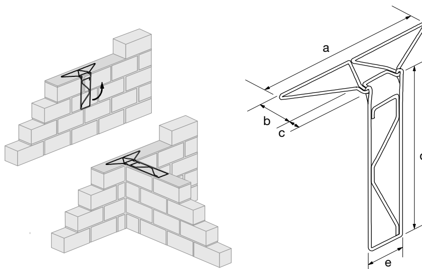
Zwischenwandanschluss KLP
