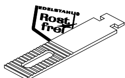
Zahnlasche Connecting plates
