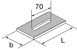
Zahnlasche Connecting plates
