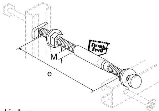
Spannverbindung
