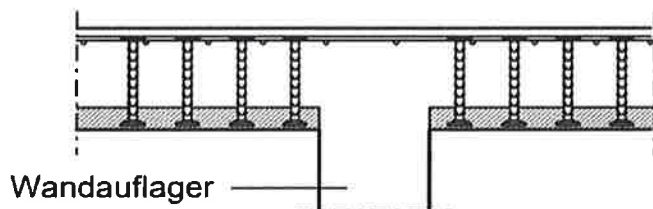
Beispiel 4: Elementdecke
