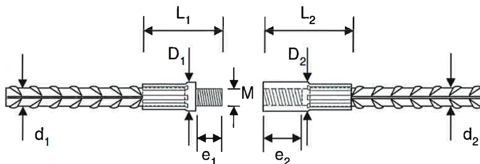
Anschlussstab BCM
