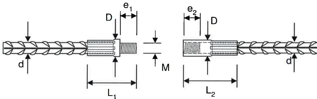
Anschlussstab BCM
