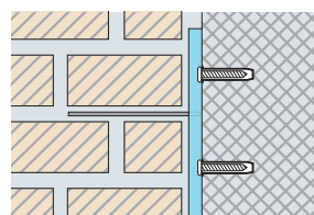
KE-Double-Joint Anchor
